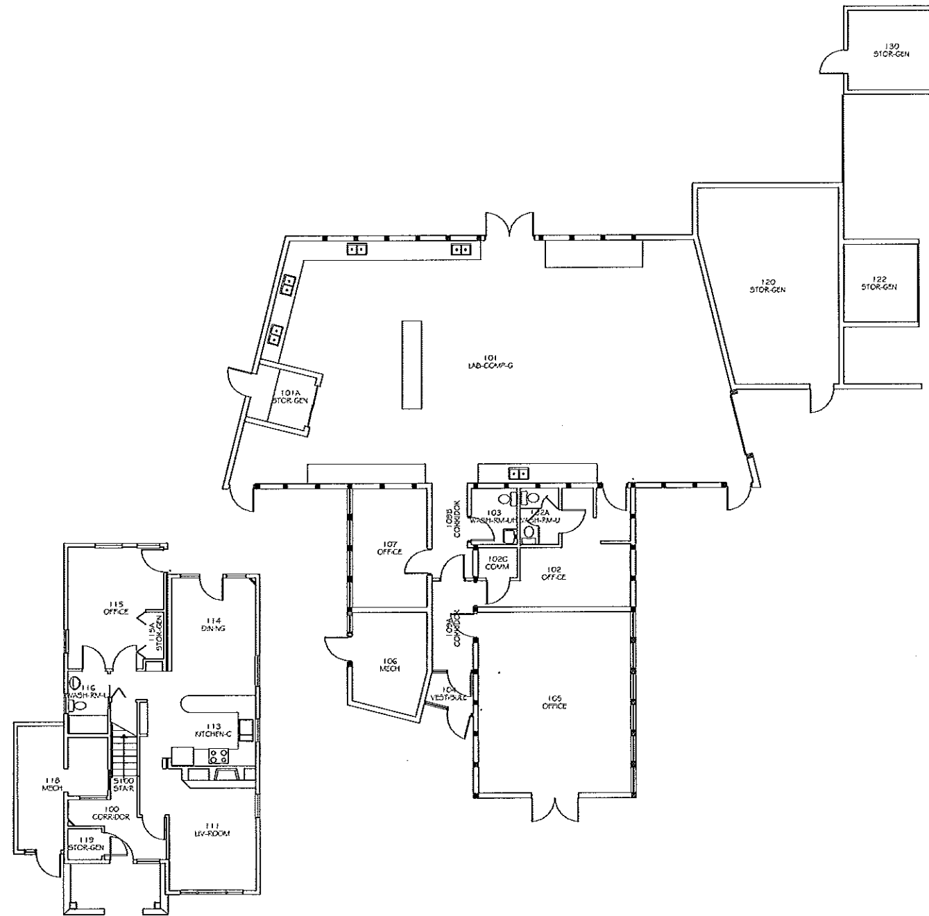
NE03, FIRST FLOOR SCALE: 1:200
